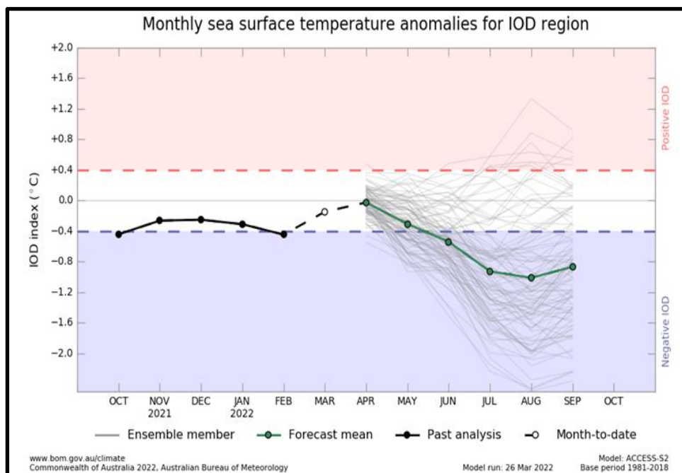
Gambar 3. Grafik DMI dari Oktober 2021 s/d September 2022
