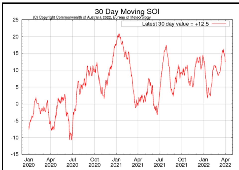
Gambar 2. Grafik SOI dari Januari 2020 s/d April 2022
