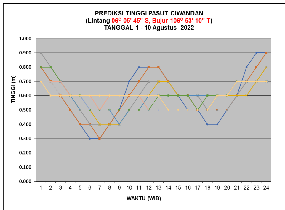
Gambar 4. Grafik Tinggi Pasang Surut Dasarian I Bulan Agustus 2022
