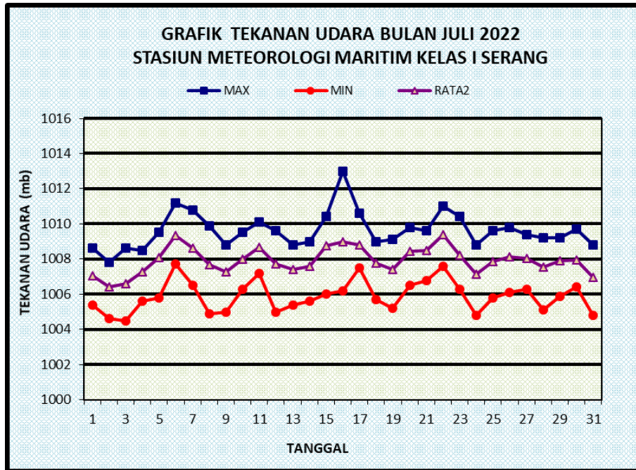
Gambar 34. Grafik Tekanan Udara
