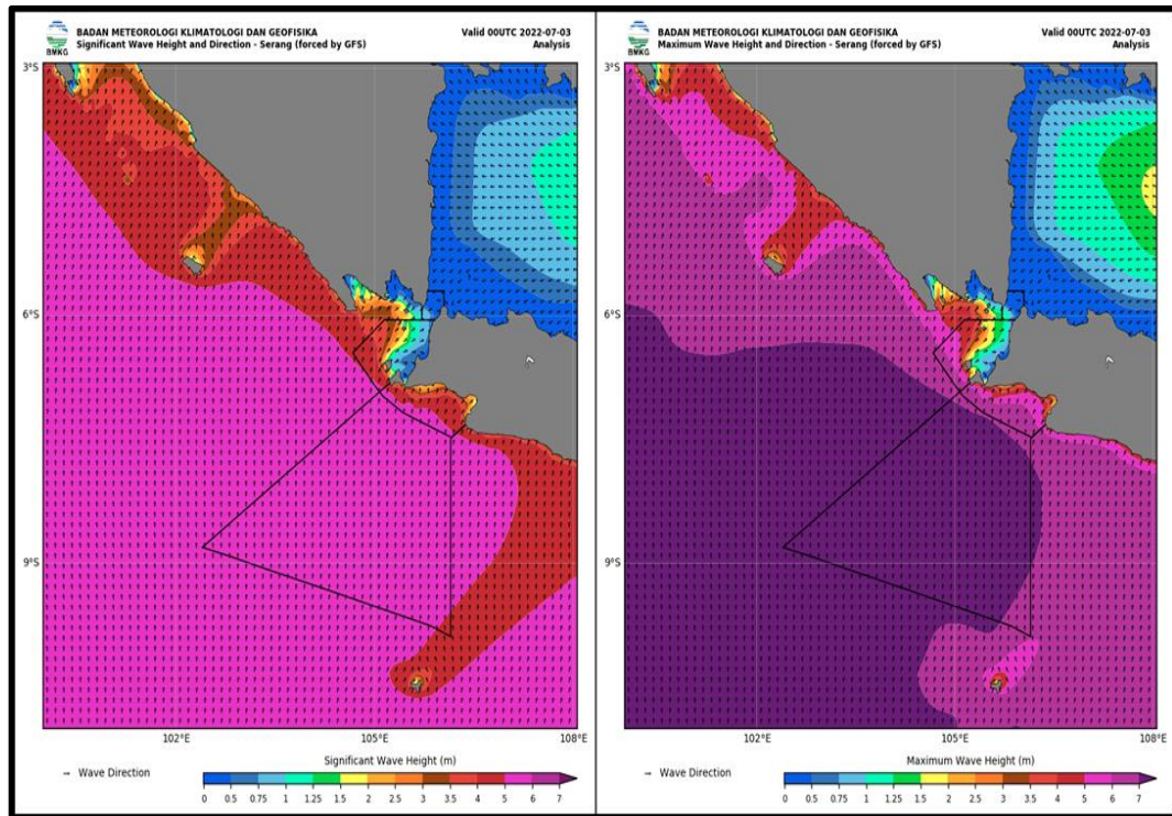
Gambar 10. Peta Analisis Tinggi Gelombang Signifikan dan Maksimum Bulan Juli 2022
