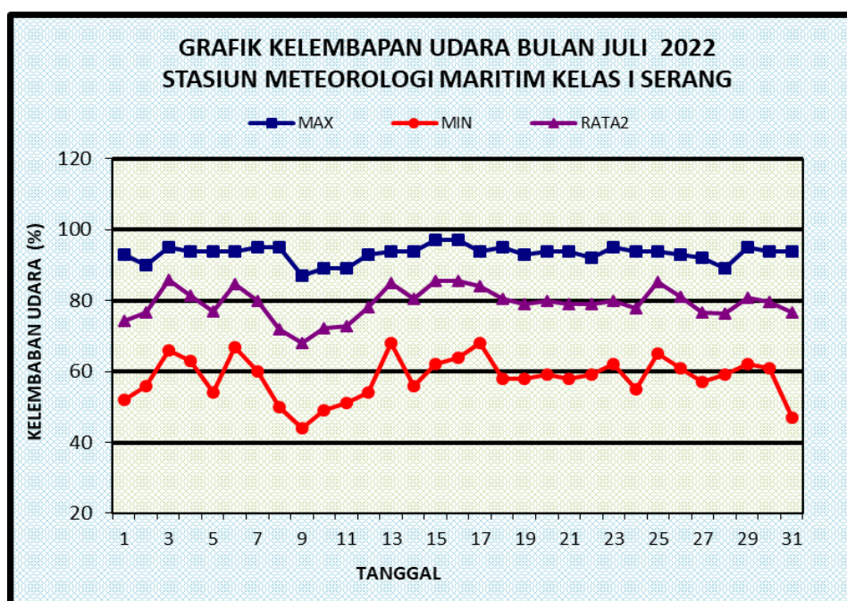
Gambar 33. Grafik Kelembapan Udara
