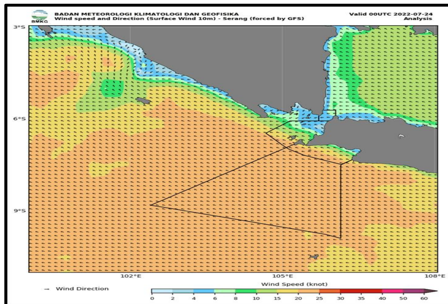
Gambar 11. Peta Analisis Arah dan Kecepatan Angin Bulan Juli 2022
