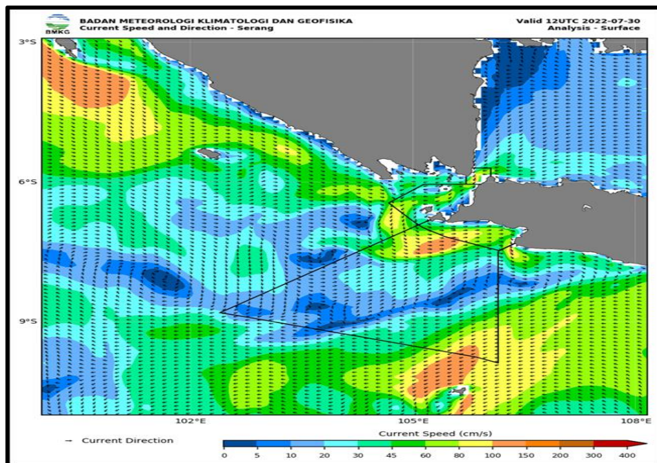
Gambar 12. Peta Analisis Arah dan Kecepatan Arus Laut Bulan Juli 2022
