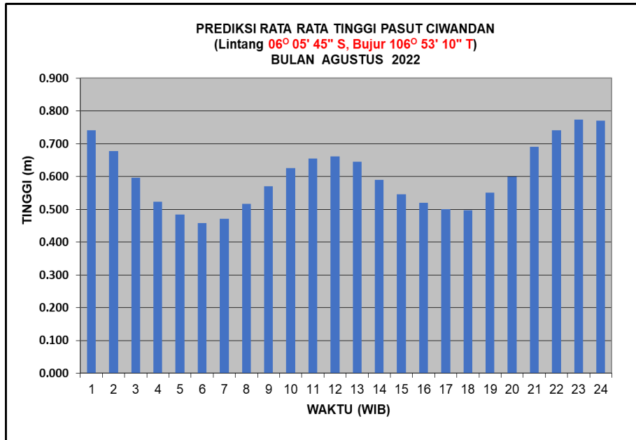
Gambar 7. Grafik Prediksi Rata-rata Tinggi Pasang Surut Bulan Agustus 2022
