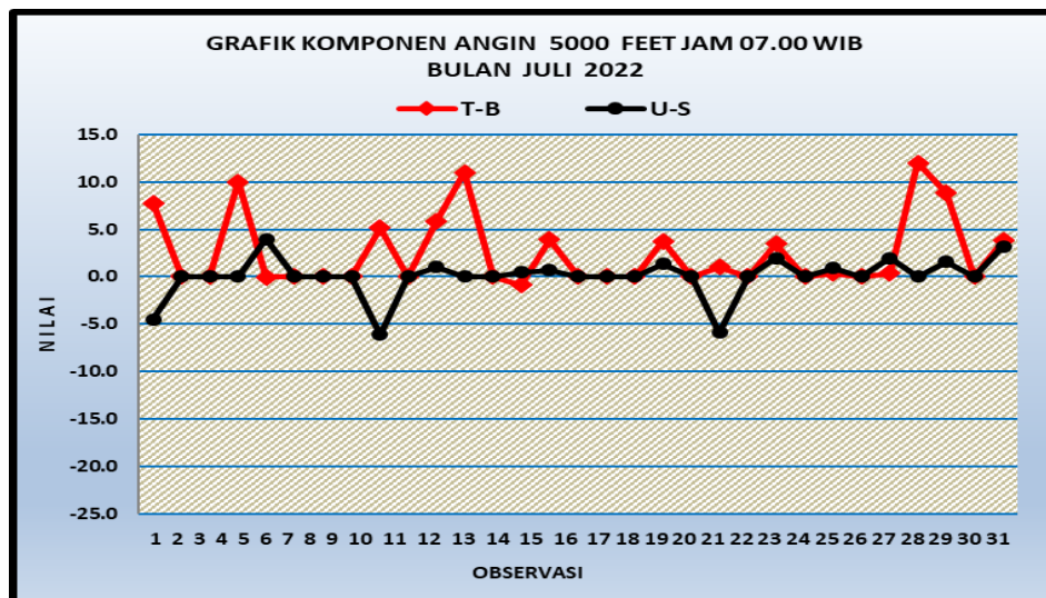
Gambar 25. Grafik komponen angin lapisan 5000 feet jam 07.00 WIB
