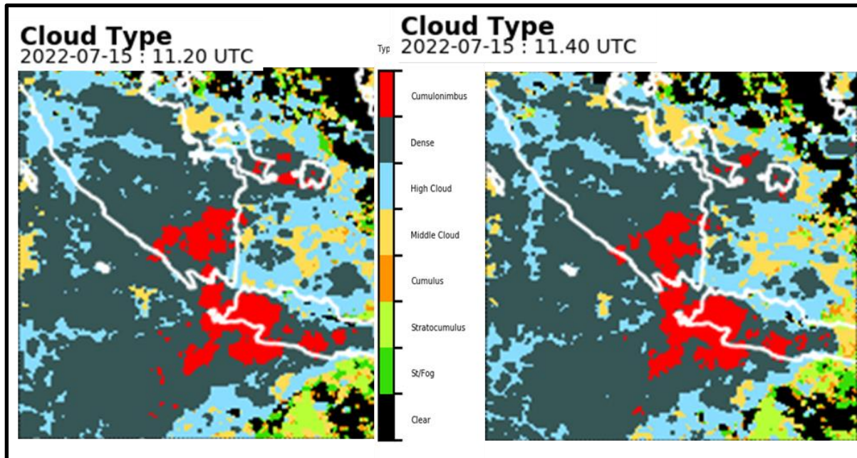
Gambar 31. Citra Satelit Himawari-8 produk Cloud Type Tanggal 15 Juli 2022 Pukul 18.20 WIB dan 18.40 WIB (Sumber : ftp://172.19.2.45 )
