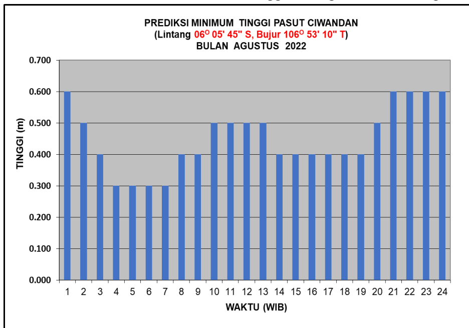
Gambar 8. Grafik Prediksi Minimum Tinggi Pasang Surut Bulan Agustus 2022
