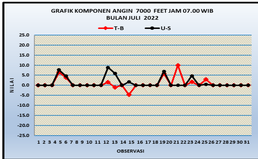
Gambar 26. Grafik komponen angin lapisan 7000 feet jam 07.00 WIB
