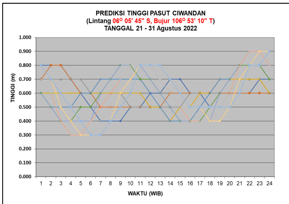
Gambar 6. Grafik Tinggi Pasang Surut Dasarian III Bulan Agustus 2022
