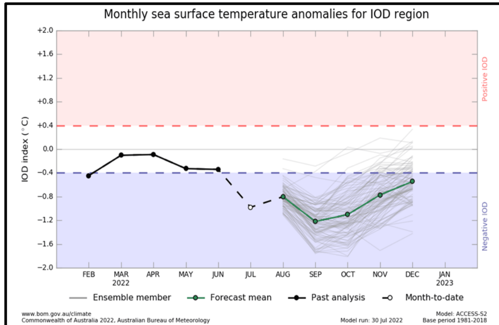
Gambar 3. Grafik DMI dari Februari 2022 s/d Desember 2022
