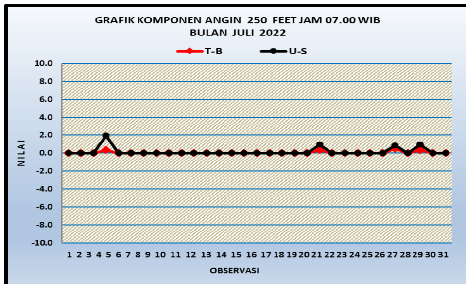
Gambar 22. Grafik komponen angin lapisan 250 feet jam 07.00 WIB
