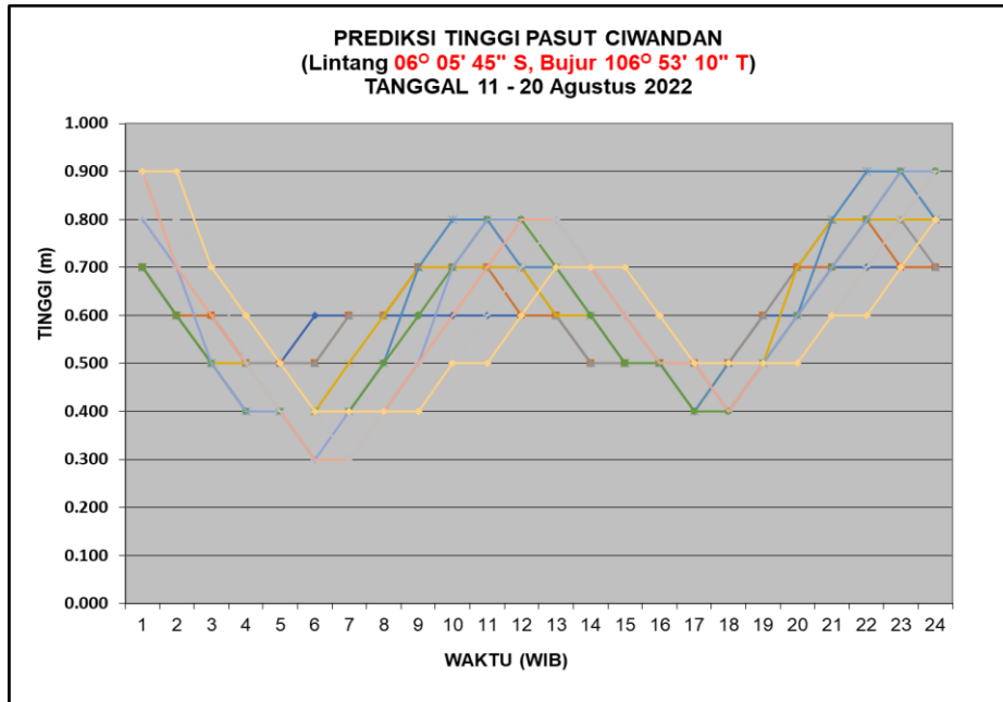
Gambar 5. Grafik Tinggi Pasang Surut Dasarian II Bulan Agustus 2022
