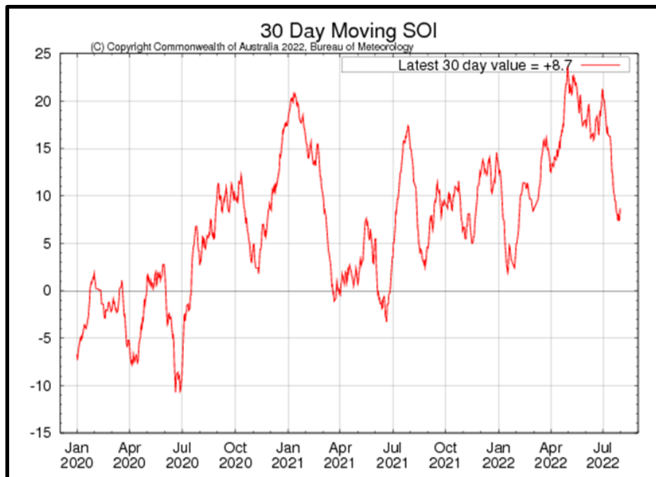
Gambar 2. Grafik SOI dari Januari 2020 s/d Agustus 2022
