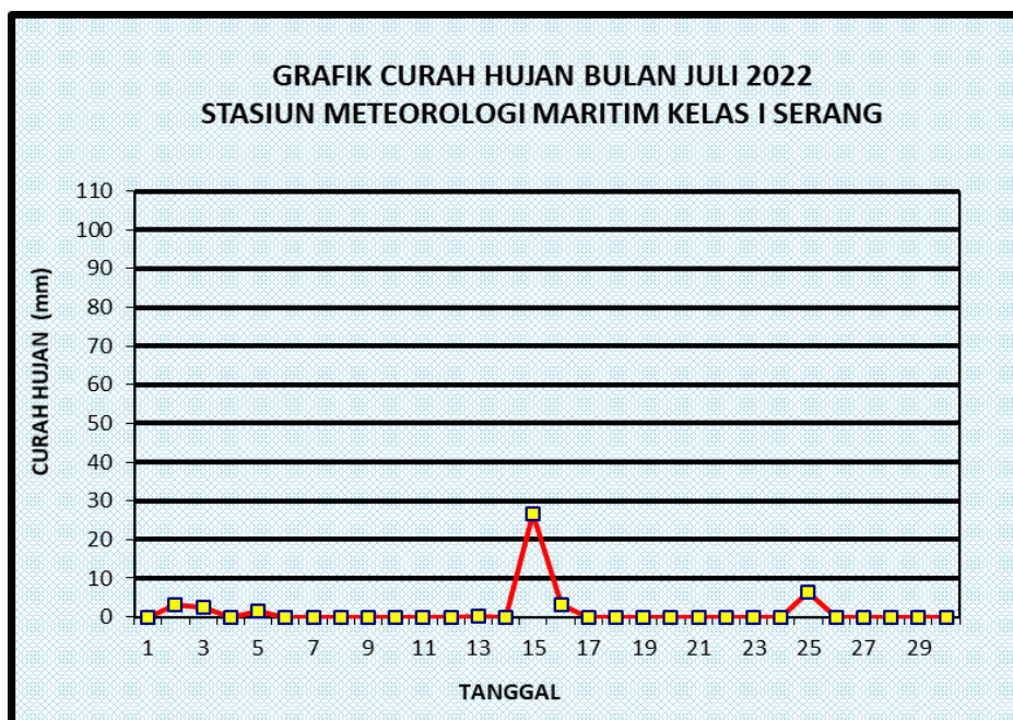
Gambar 35. Grafik Curah Hujan
