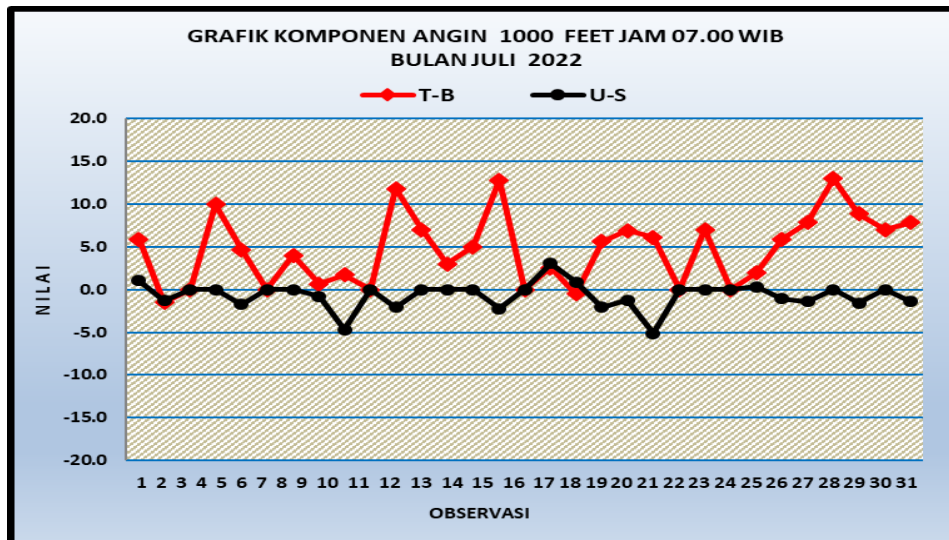
Gambar 23. Grafik komponen angin lapisan 1000 feet jam 07.00 WIB
