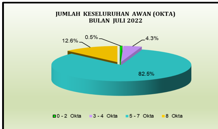
Gambar 14. Grafik Jumlah Keseluruhan Awan (okta)
