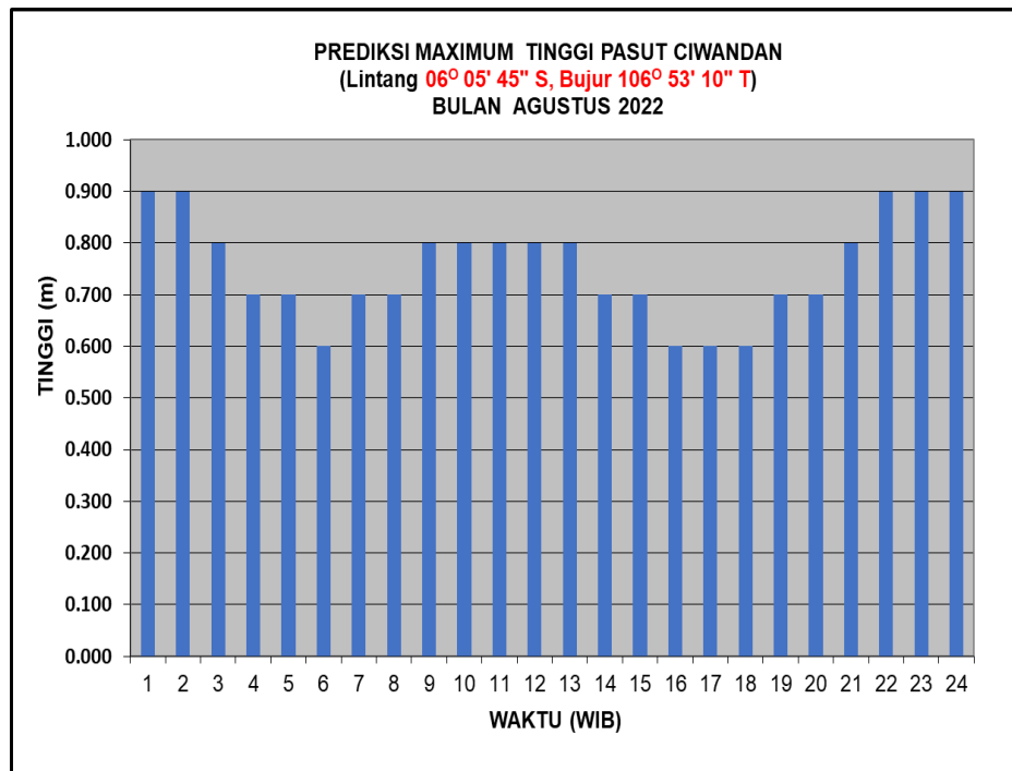
Gambar 9. Grafik Prediksi Maximum Tinggi Pasang Surut Bulan Agustus 2022
