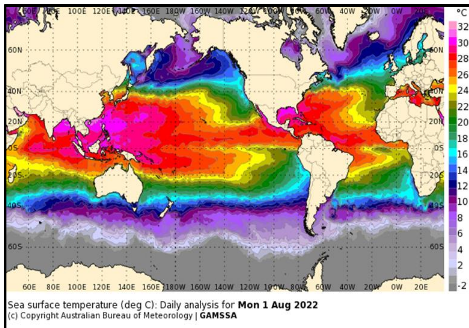
Gambar 1. Suhu muka laut (SST) Agustus 2022
