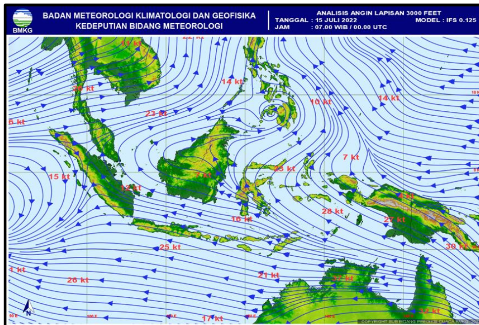
Gambar 30. Analisis Streamline pada 15 Juli 2022 jam 07.00 WIB
