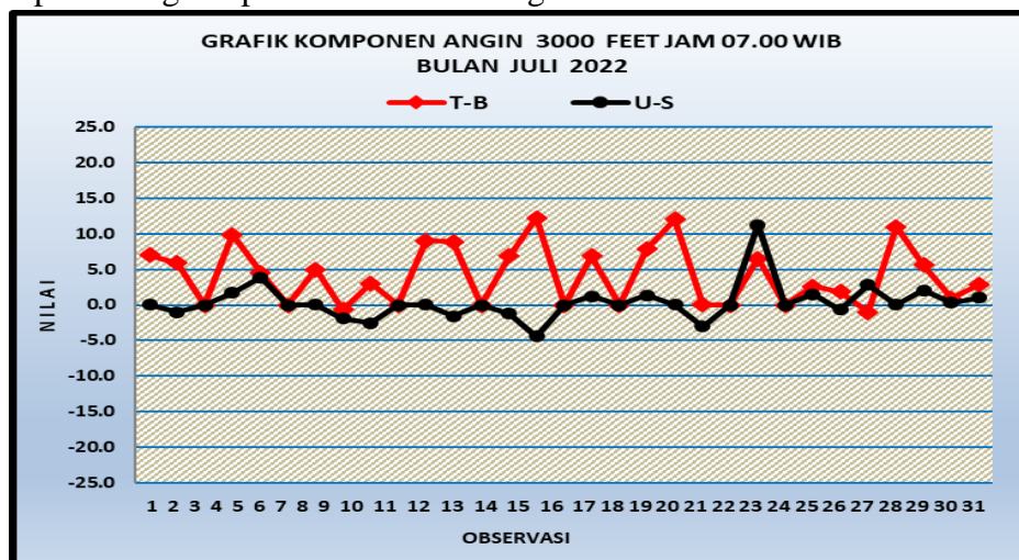
Gambar 24. Grafik komponen angin lapisan 3000 feet jam 07.00 WIB
