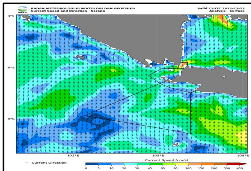
Gambar 12. Peta Analisis Arah dan Kecepatan Arus Laut Bulan Desember 2022
