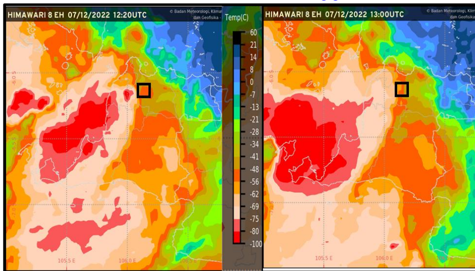
Gambar 32. Citra Satelit Himawari-8 produk Cloud Type Tanggal 7 Desember 2022 Pukul 19.20 WIB dan 20.00 WIB
