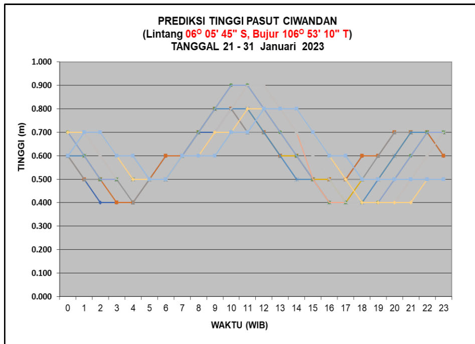
Gambar 6. GrafikTinggi Pasang Surut Dasarian III Bulan Januari 2023
