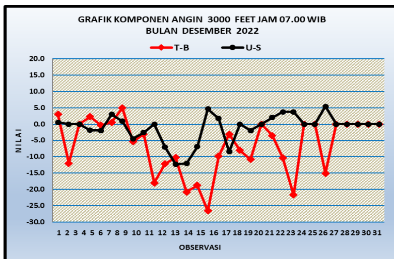
Gambar 24. Grafik komponen angin lapisan 3000 feet jam 07.00 WIB
