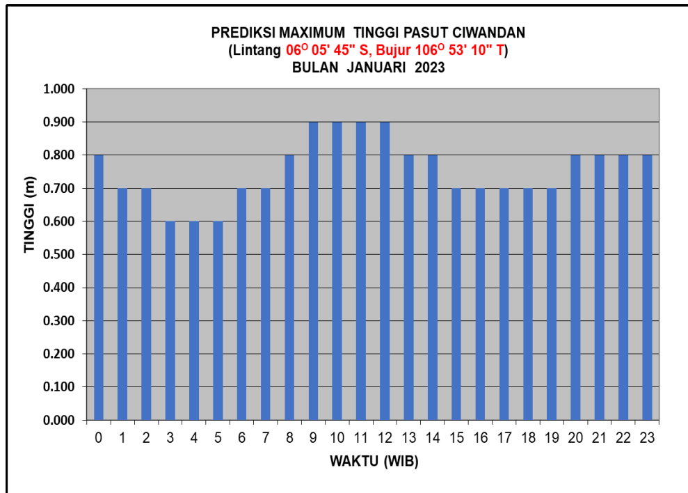
Gambar 9. Grafik Prediksi Maximum Tinggi Pasang Surut Bulan Januari 2023
