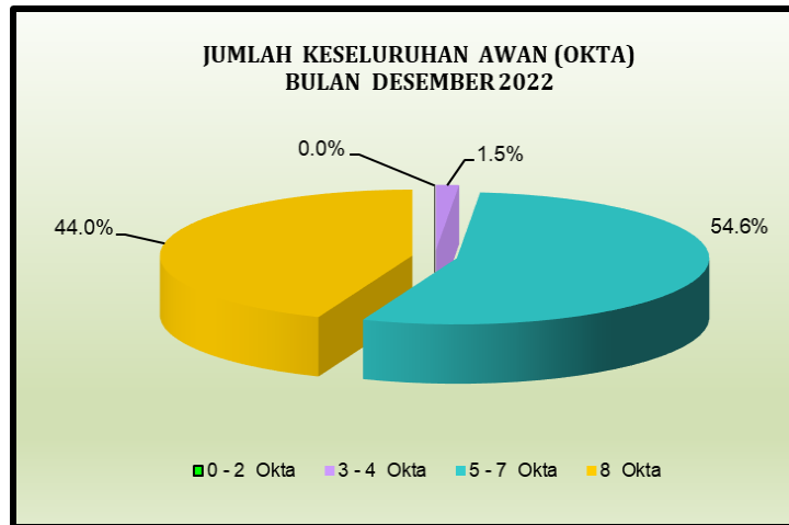
Gambar 14. Grafik Jumlah Keseluruhan Awan (okta)
