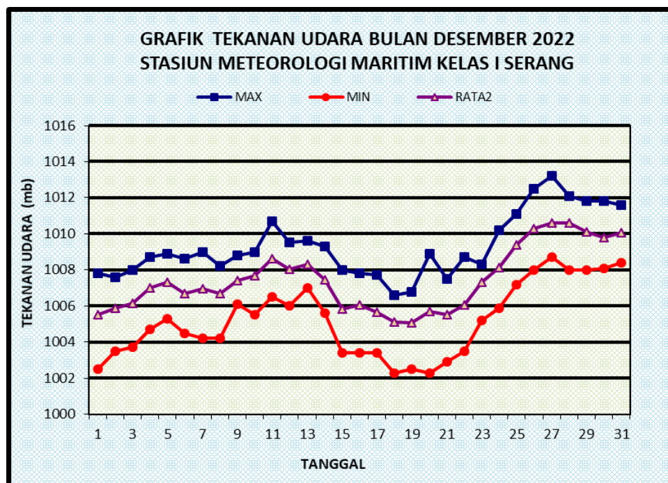
Gambar 34. Grafik Tekanan Udara
