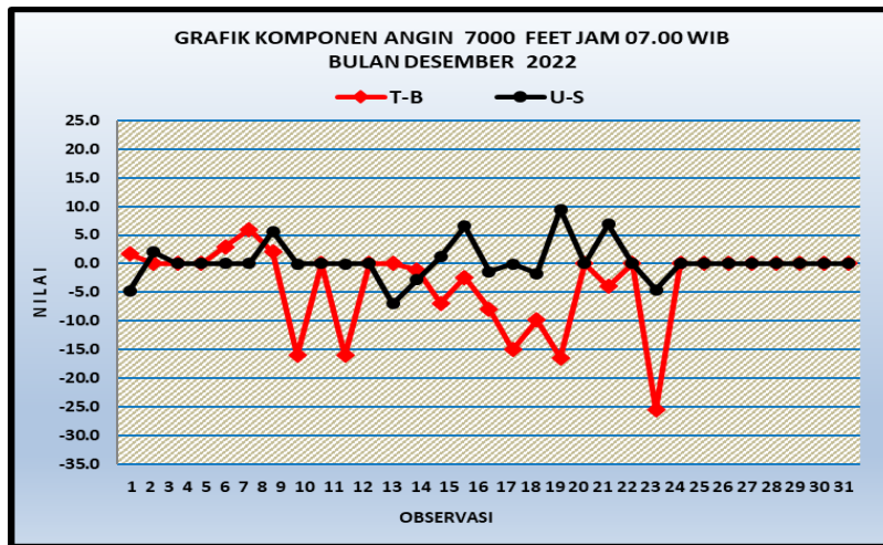
Gambar 26. Grafik komponen angin lapisan 7000 feet jam 07.00 WIB
