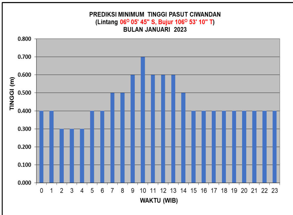
Gambar 8. Grafik Prediksi Minimum Tinggi Pasang Surut Bulan Januari 2023
