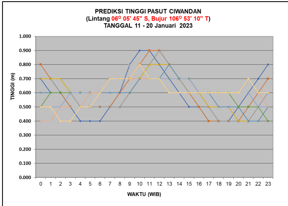
Gambar 5. GrafikTinggi Pasang Surut Dasarian II Bulan Januari 2023
