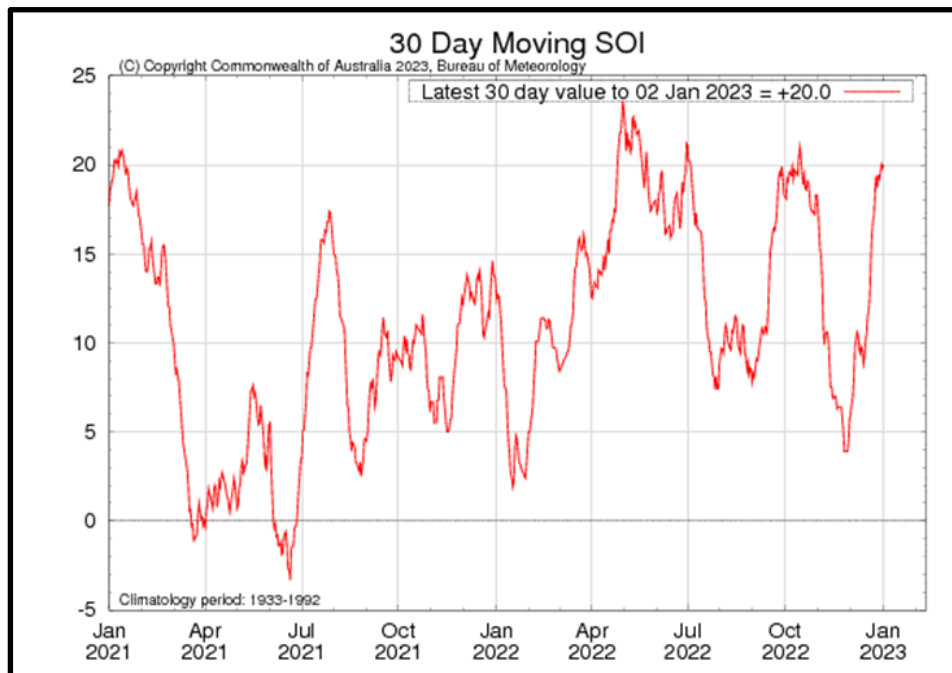
Gambar 2. Grafik SOI dari Januari 2021 s/d Januari 2023
