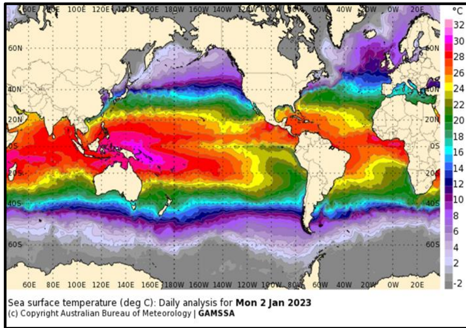
Gambar 1. Suhu muka laut (SST) Januari 2023
