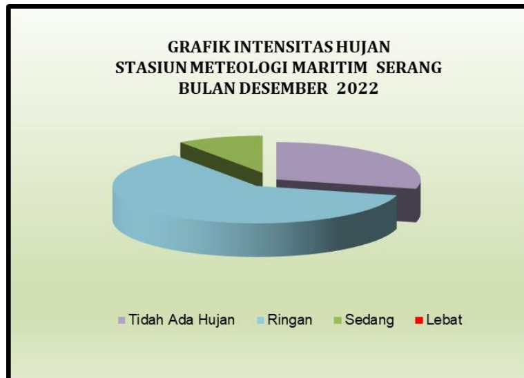
Gambar 13. Grafik Intensitas Hujan
