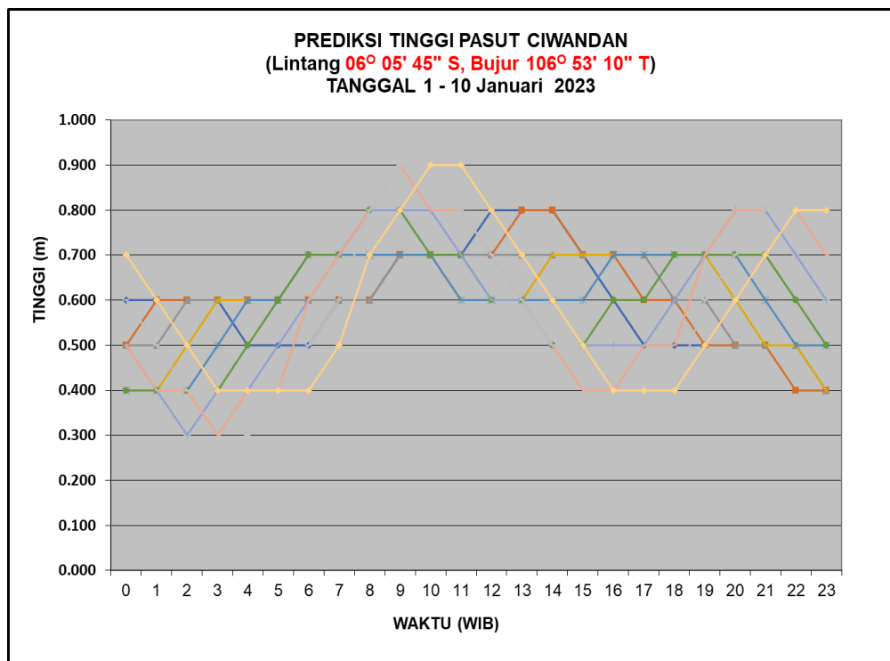
Gambar 4. Grafik Tinggi Pasang Surut Dasarian I Bulan Januari 2023
