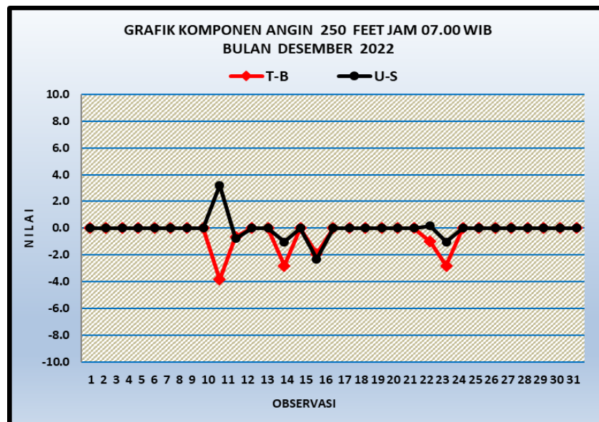
Gambar 22. Grafik komponen angin lapisan 250 feet jam 07.00 WIB
