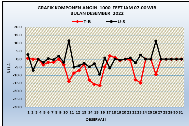
Gambar 23. Grafik komponen angin lapisan 1000 feet jam 07.00 WIB
