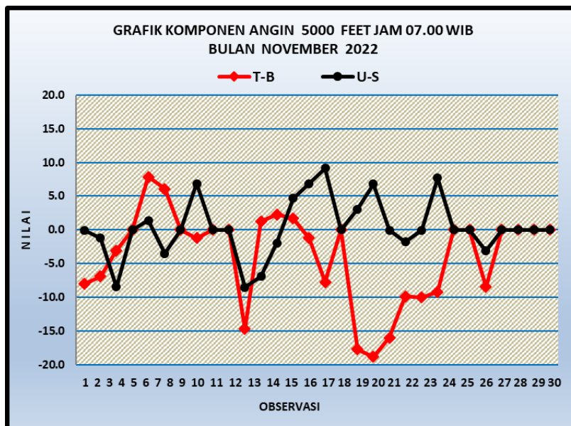
Gambar 25. Grafik komponen angin lapisan 5000 feet jam 07.00 WIB
