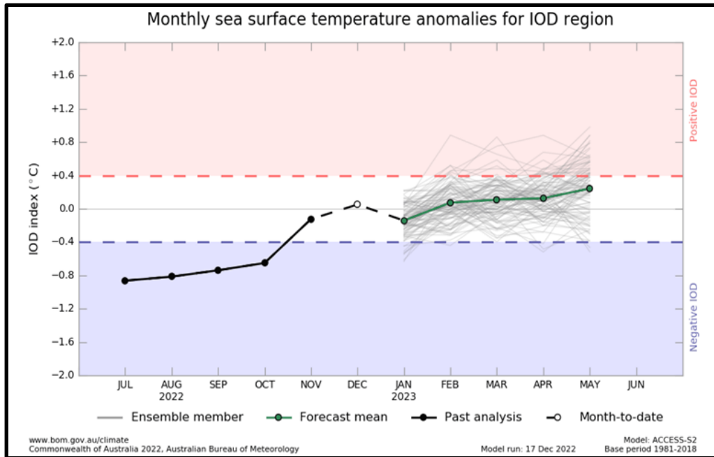
Gambar 3. Grafik DMI dari Juli 2022 s/d Mei 2023
