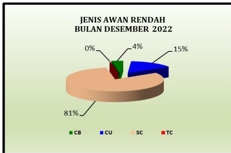
Gambar 15. Grafik Jenis Awan Rendah
