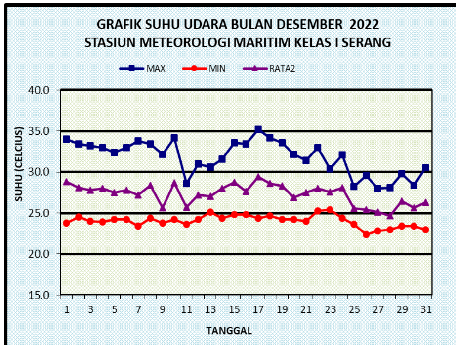
Gambar 33. Grafik Suhu Udara
