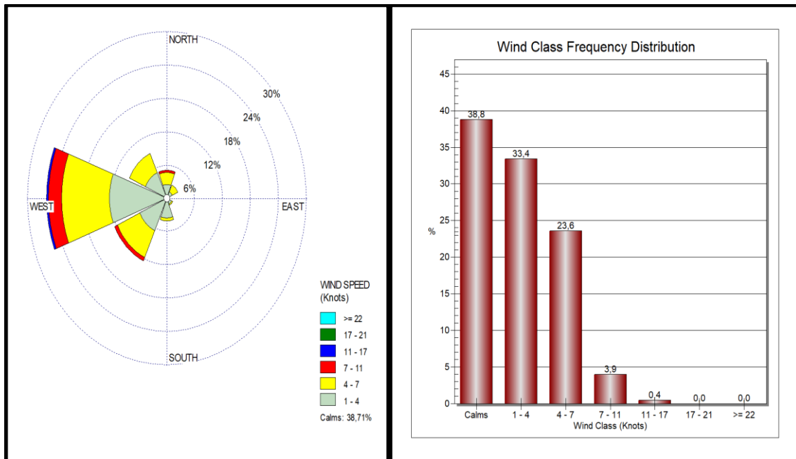
Gambar 18. Wind Rose dan klasifikasi kecepatan angin permukaan Wilayah Serang
