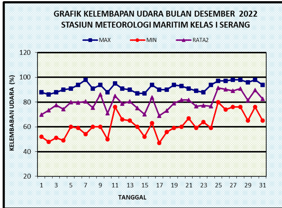
Gambar 34. Grafik Kelembapan Udara
