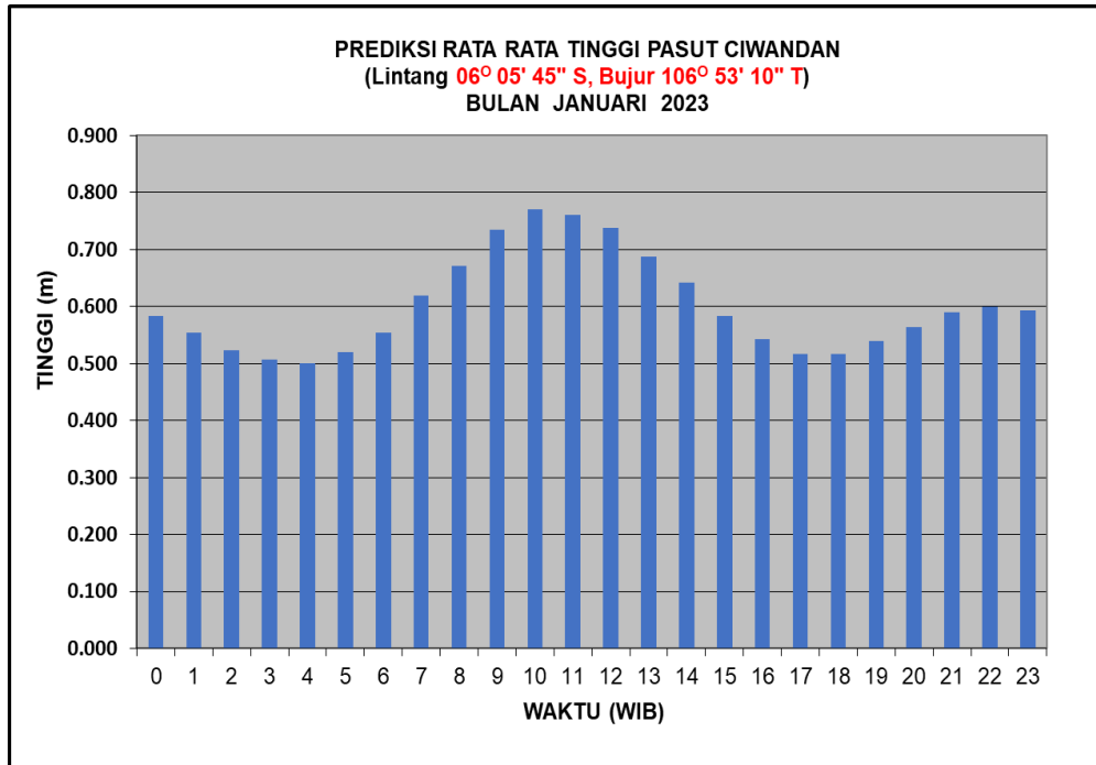
Gambar 7. Grafik Prediksi Rata-rata Tinggi Pasang Surut Bulan Januari 2023
