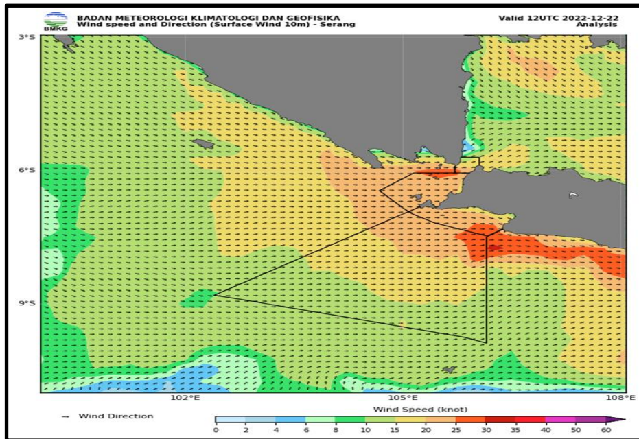
Gambar 11. Peta Analisis Arah dan Kecepatan Angin Bulan Desember 2022
