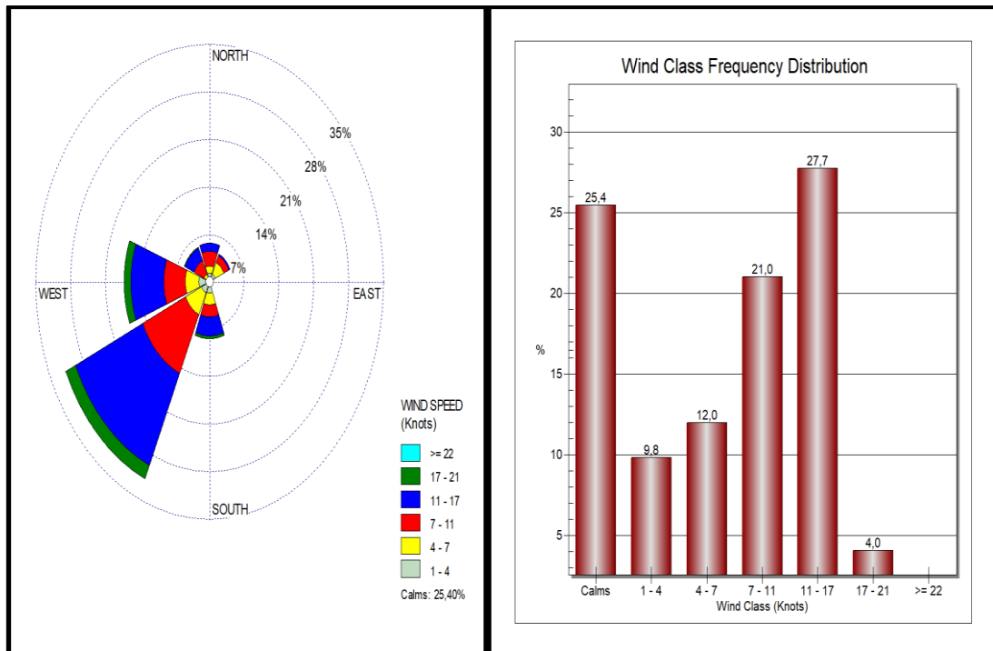
Gambar 20. Wind Rose dan klasifikasi kecepatan Permukaan Wilayah Bakauheni
