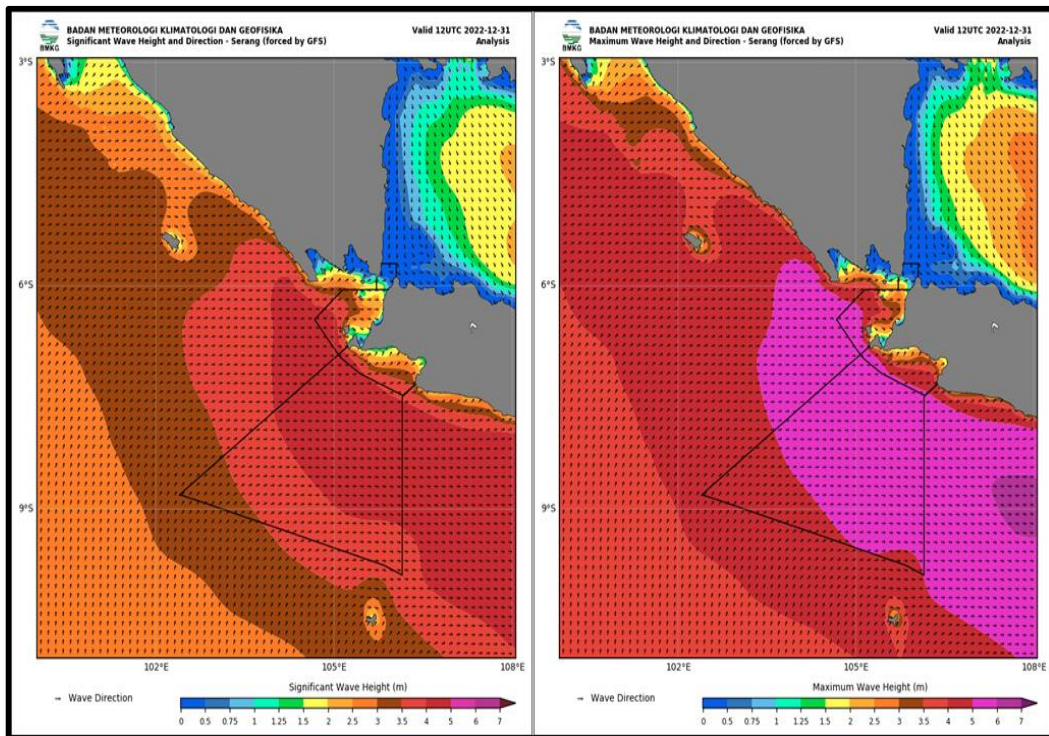
Gambar 10. Peta Analisis Tinggi Gelombang Signifikan dan Maksimum Bulan Desember 2022
